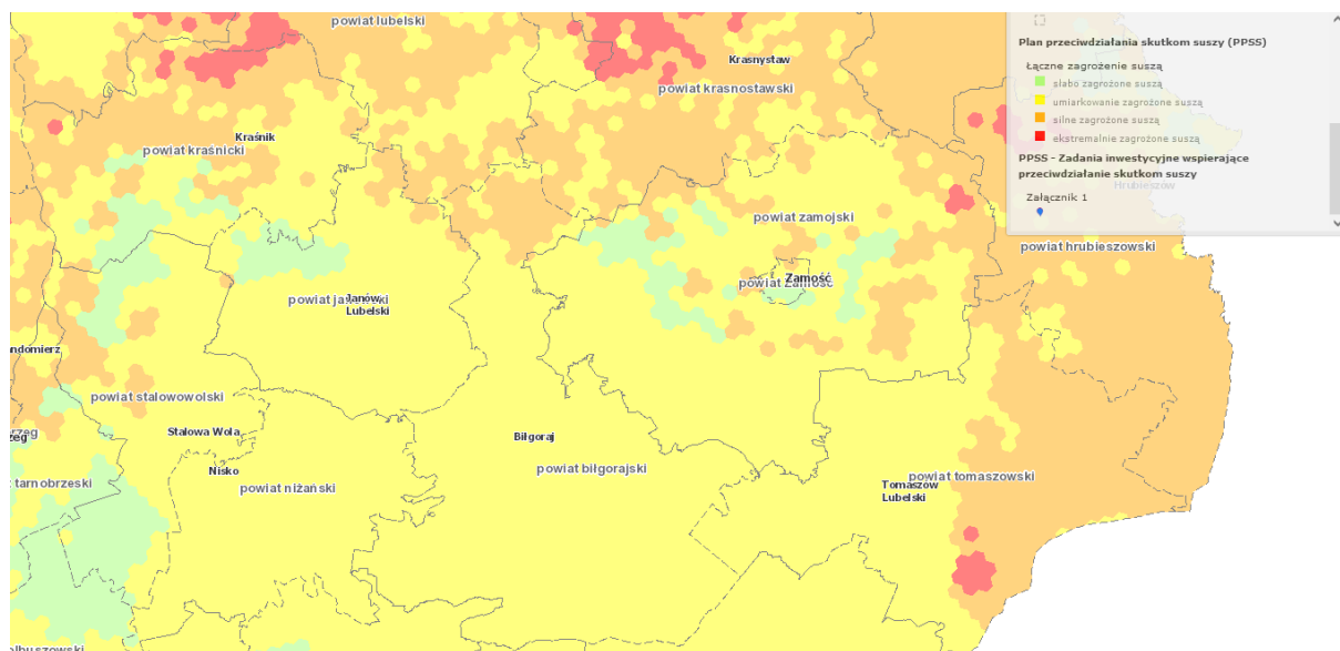
Grafika 11: Mapa zagrożeń suszą
